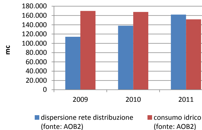
Confronto dispersione rete di distribuzione e consumo idrici (fonte: AOB2)
