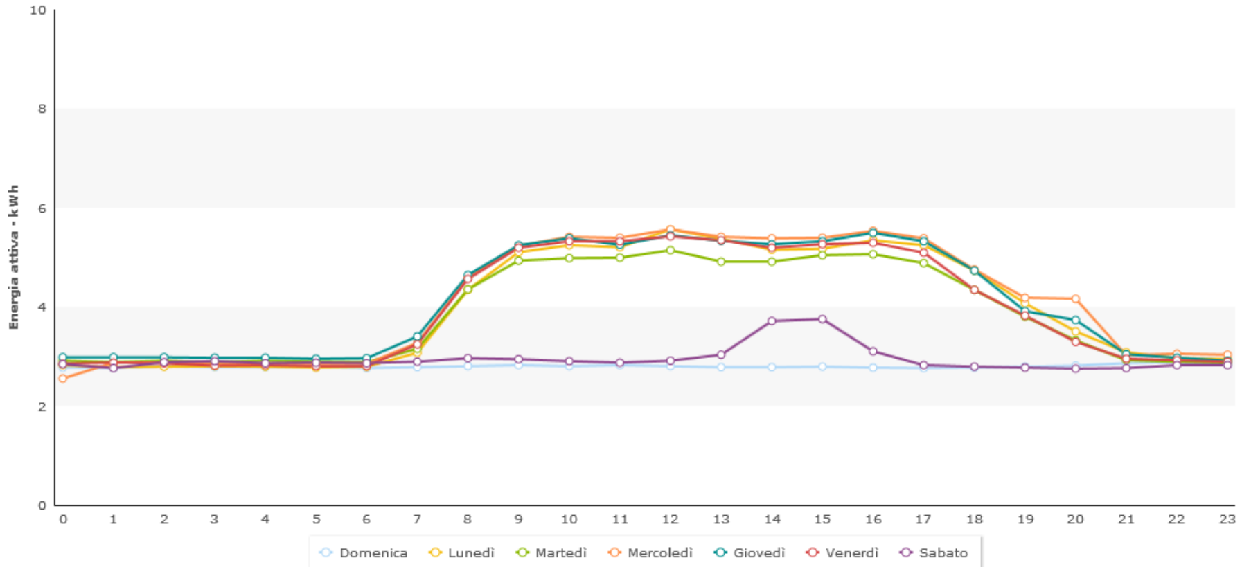
Curve di carico
